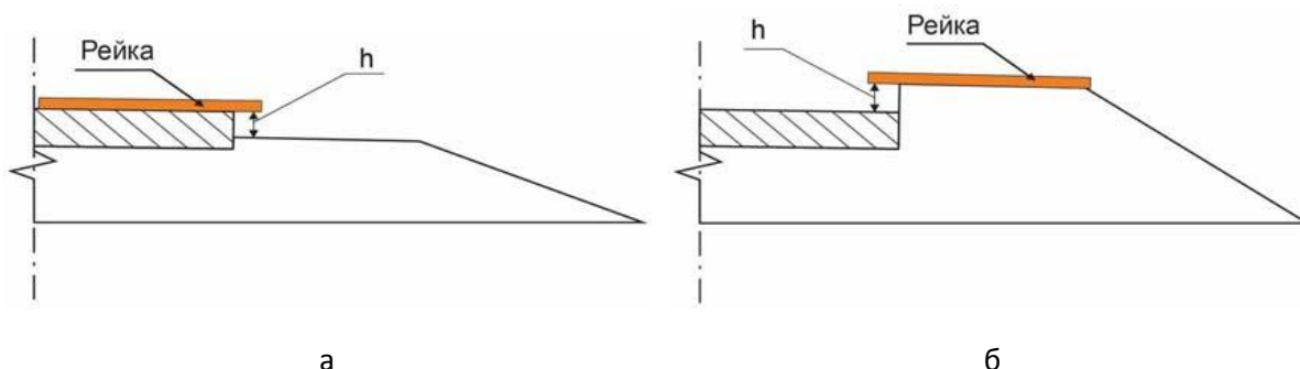
Рисунок 1 - Схема измерения величины занижения (возвышения) обочины и разделительной полосы: а - при занижении; б - при возвышении
